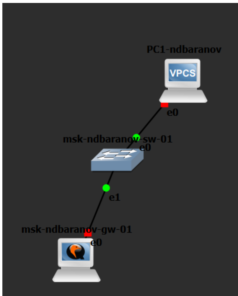
Рисунок 1 — На схеме PC1 соединён через коммутатор с маршрутизатором VyOS
