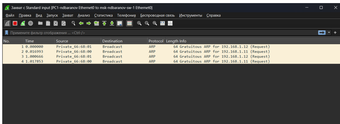
Рисунок 4.6: В списке Wireshark видны широковещательные ARP-запросы о владельце 192
