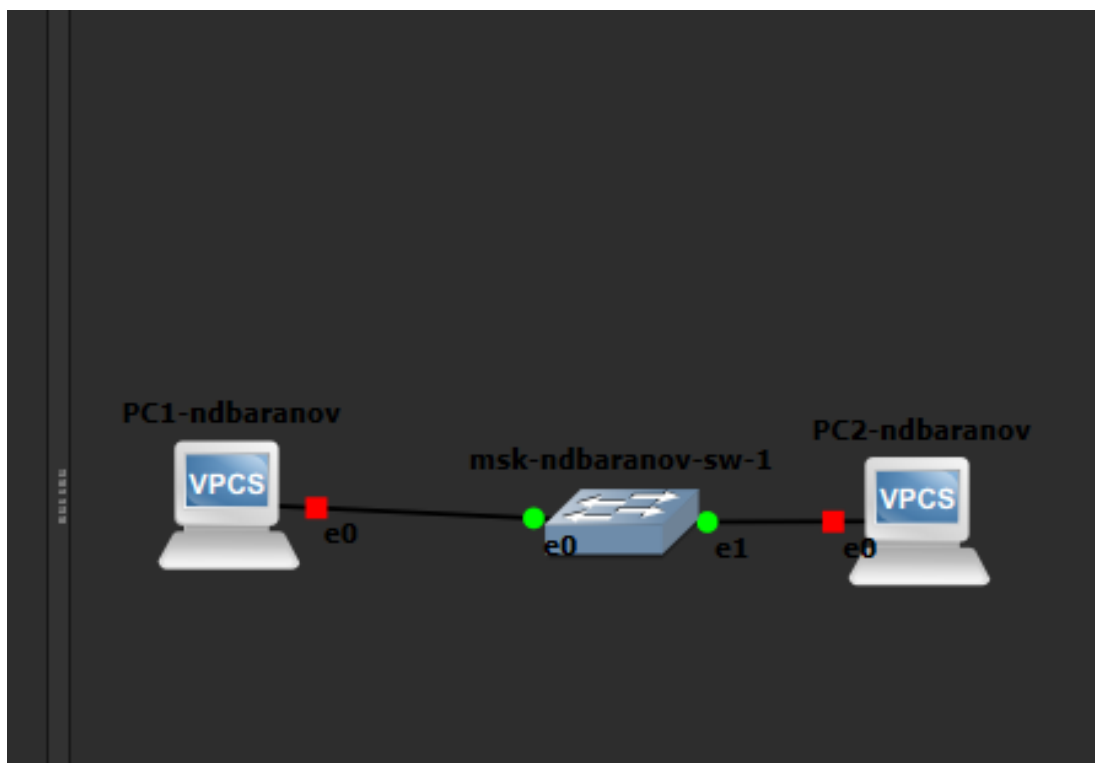
Рисунок 4.1: В GNS3 собрана минимальная локальная сеть: два узла VPCS подключены к одному Ethernet-коммутатору
