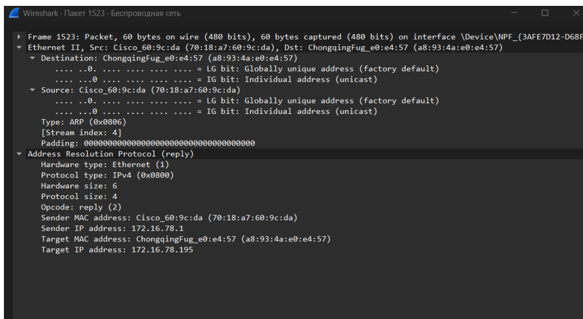
Рисунок 9 — В ARP Reply opcode изменён на reply, а поля sender содержат найденное соответствие IPv4 и MAC
