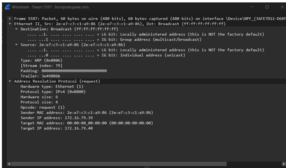
Рисунок 8 — Детали ARP Request содержат opcode request, sender MAC/IP и target IP при нулевом target MAC
