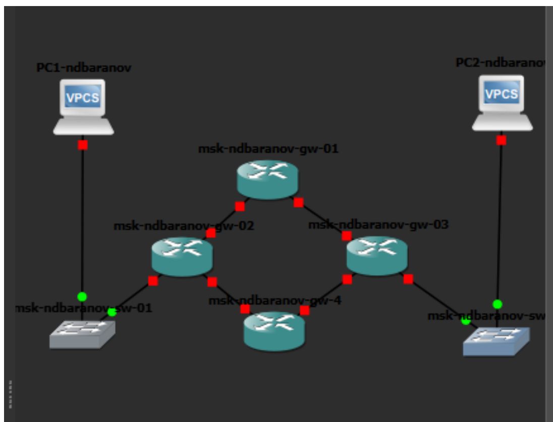
Рисунок 4.1: В GNS3 построено кольцо из четырёх маршрутизаторов FRR с двумя конечными сетями
