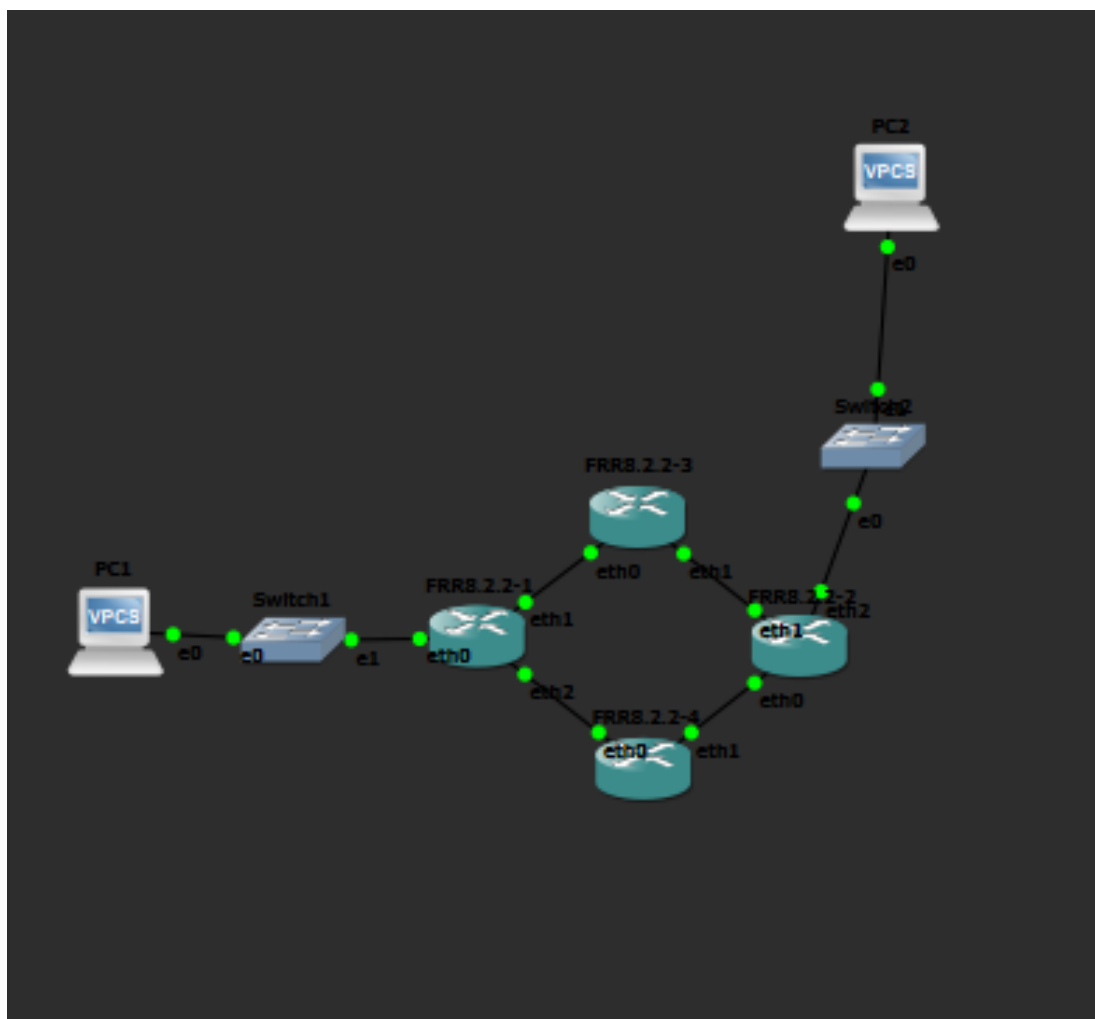
Рисунок 4.20: После запуска маршрутизации рабочая схема показана с зелёными соединениями по основным и резервным путям
