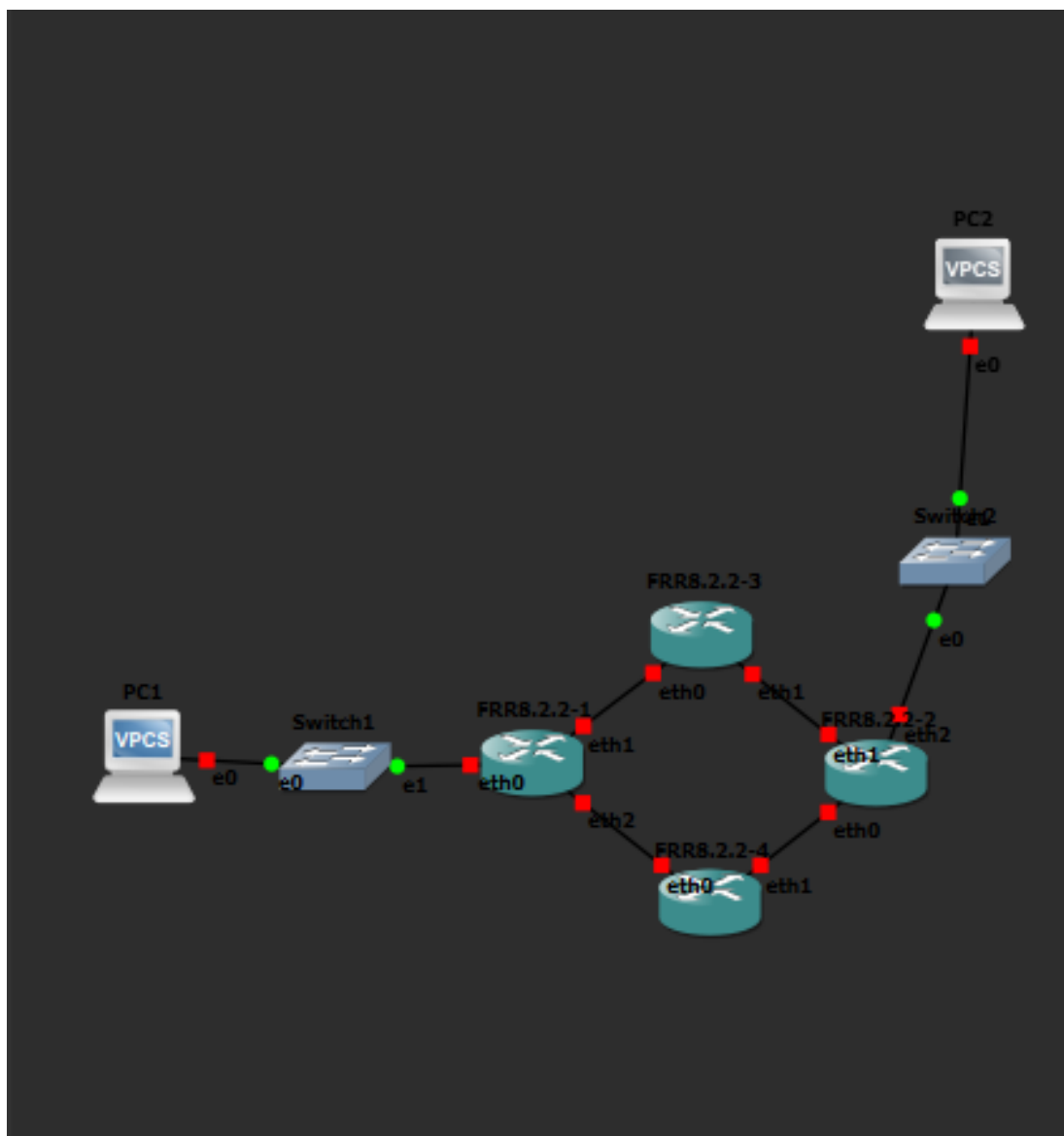
Рисунок 4.16: Для самостоятельного варианта собрана топология с четырьмя FRR и двумя VPCS, где между частью маршрутизаторов существуют резервные линии
