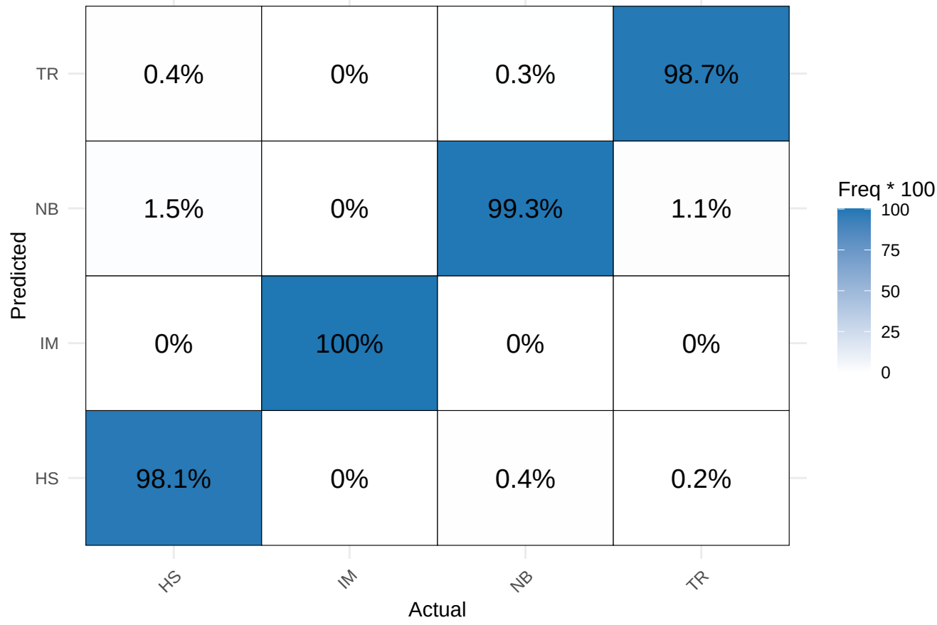
Confusion Matrix: MLP-ML
