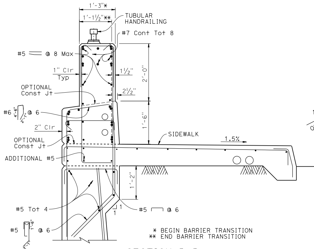
SECTION D-D
