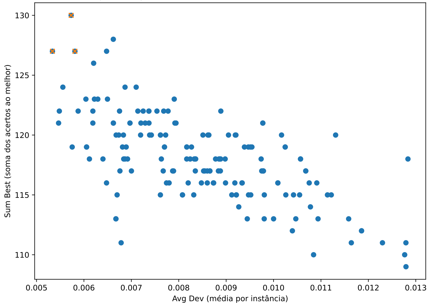
GA — Ajuste de parâmetros (selecionadas destacadas, instâncias 1-16)
