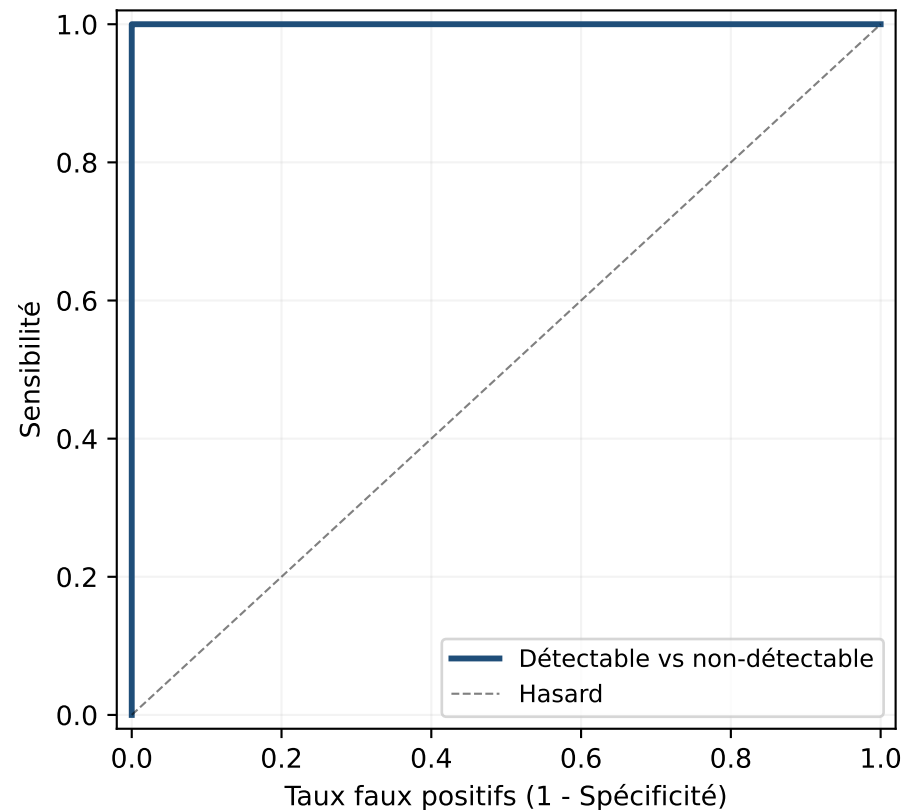
(a) Séparabilité détectable vs non-détectable AUC = 1.000 [IC95 : 1.000, 1.000]
