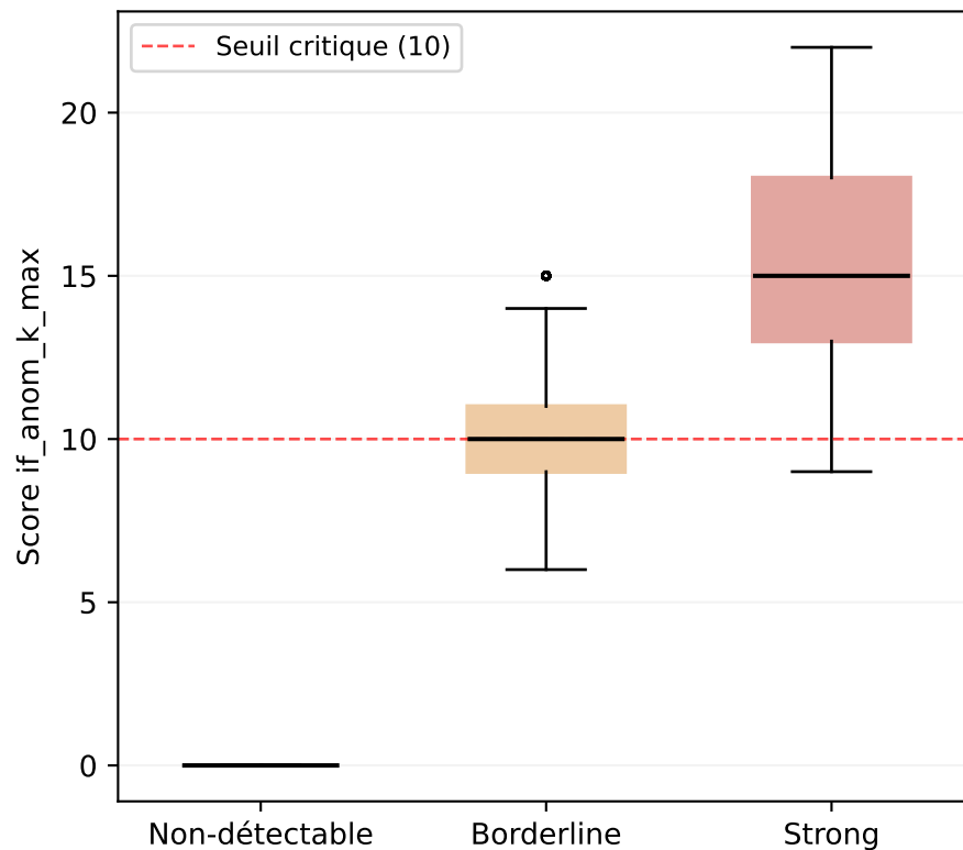
(b) Distribution du score par profil (18 816 événements)
