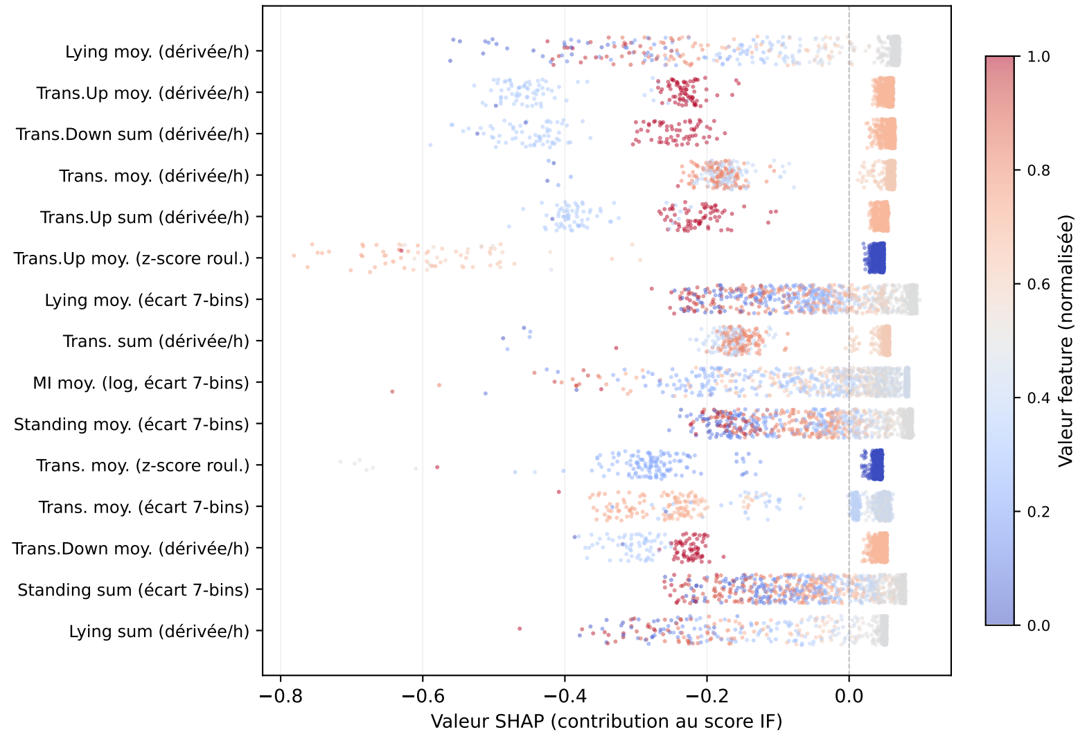
(b) Distribution des contributions (couleur = valeur feature)
