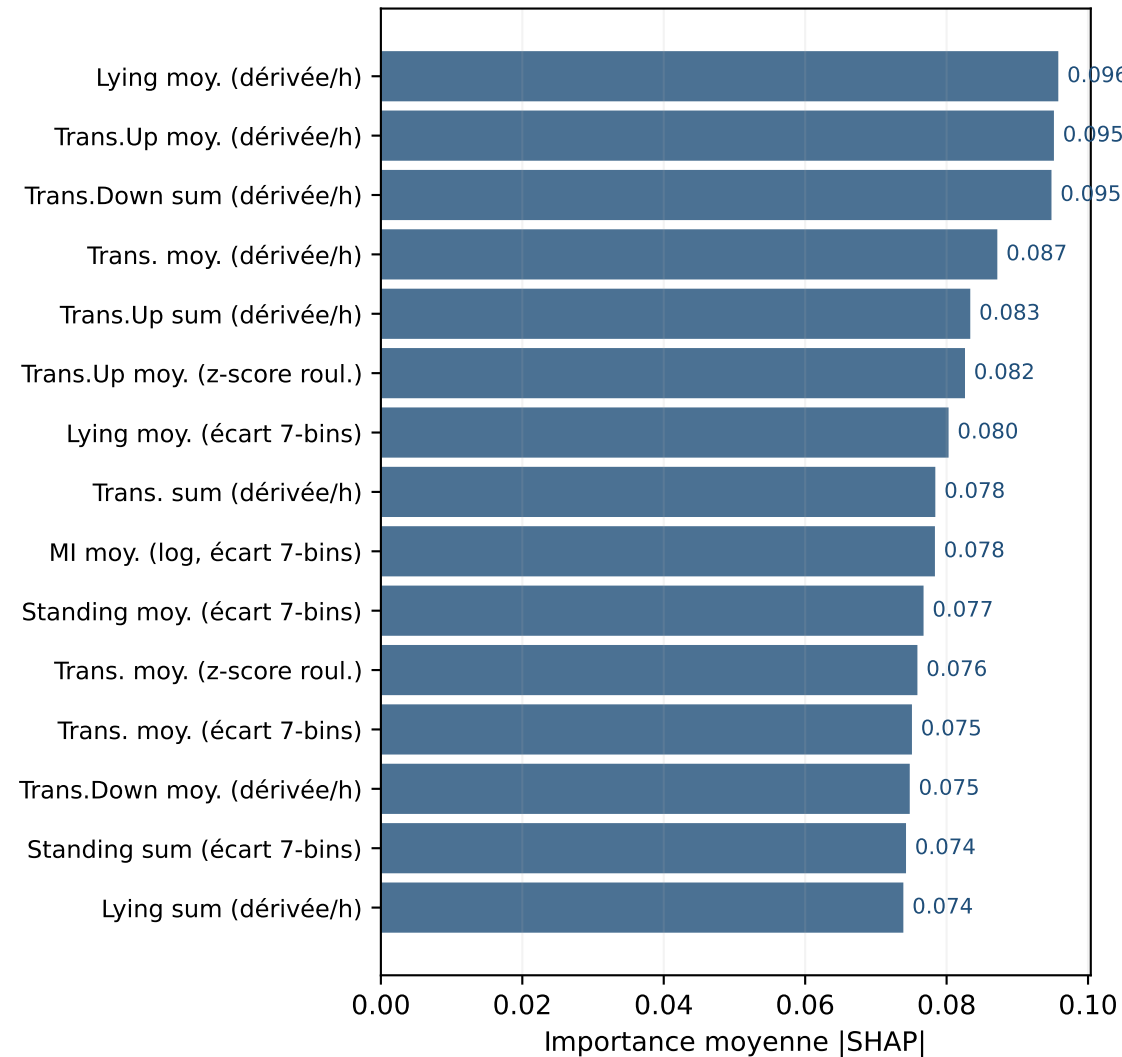
(a) Top 15 features par importance globale
