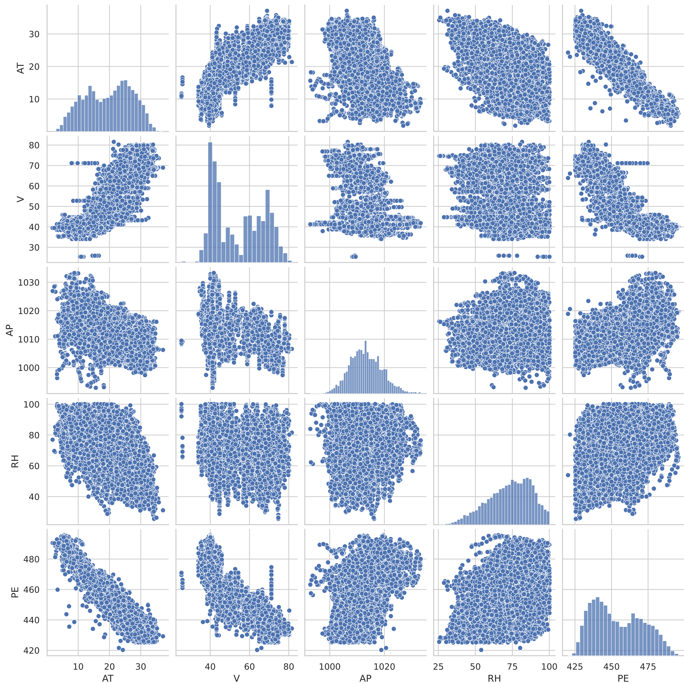
Pairwise Scatterplots
