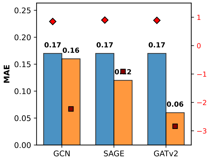
Skew MAE
