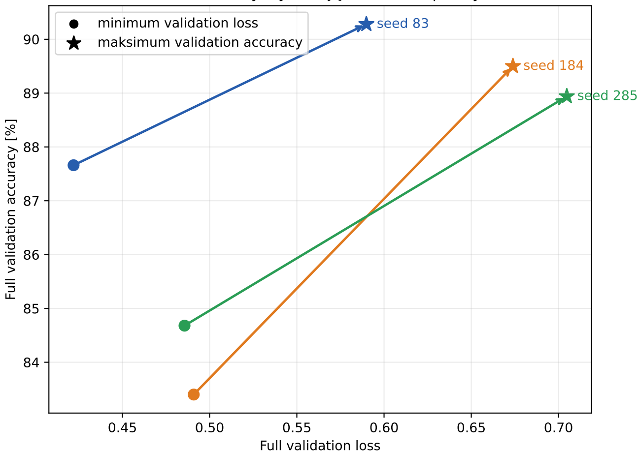
P1=1: loss i accuracy wybierają inne checkpointy Phase 2
