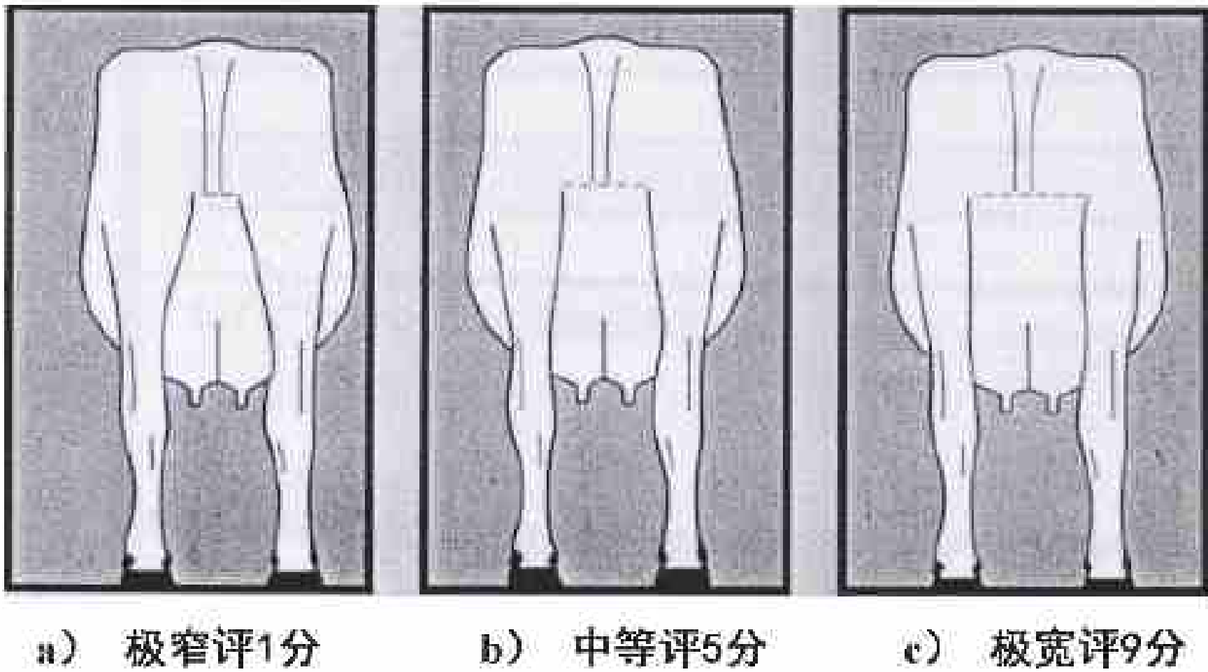
图 C.18 后乳房附着宽度评分示意图
