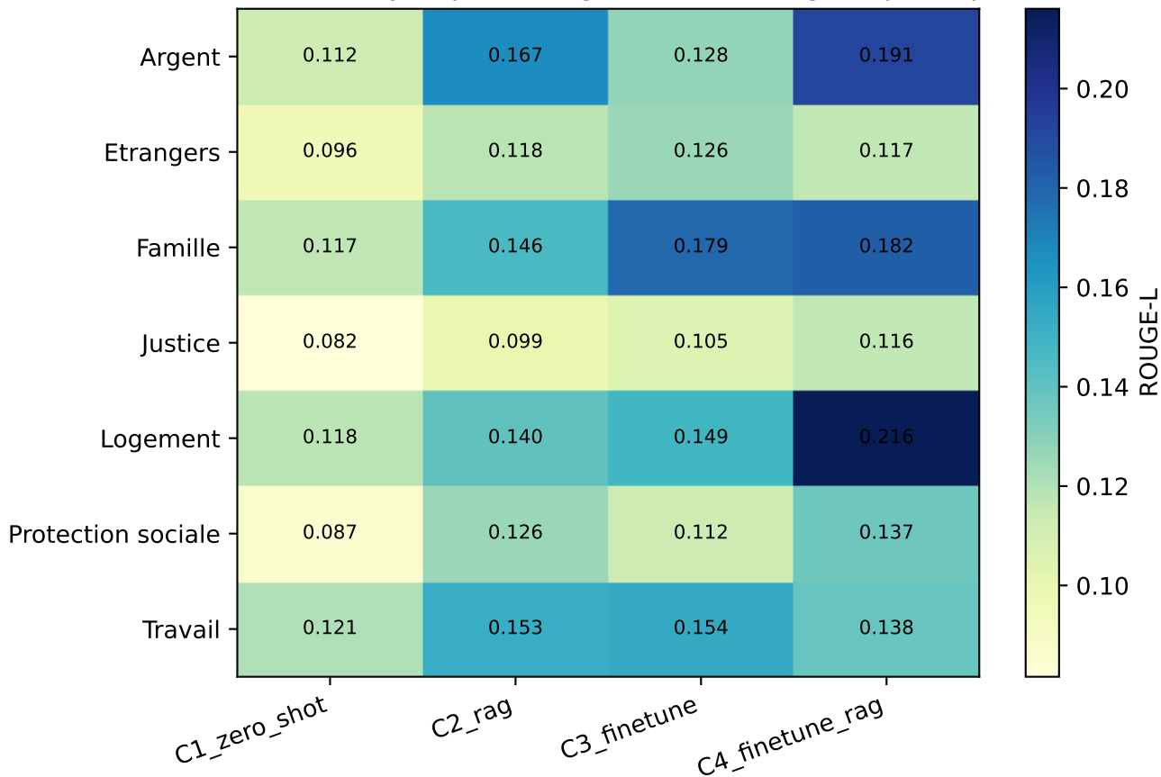
ROUGE-L moyen par configuration × catégorie juridique
