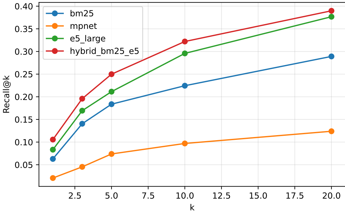
Recall@k par méthode de retrieval (222 questions test)
