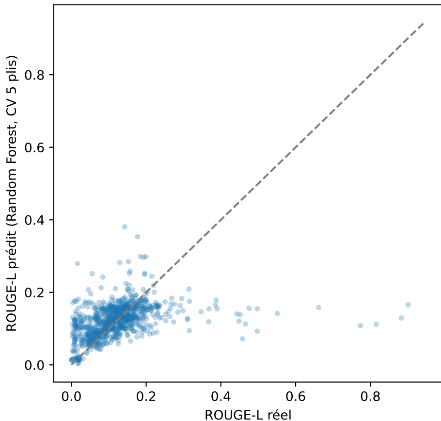
Prédit vs réel — ROUGE-L ( R^2=0.132 )
