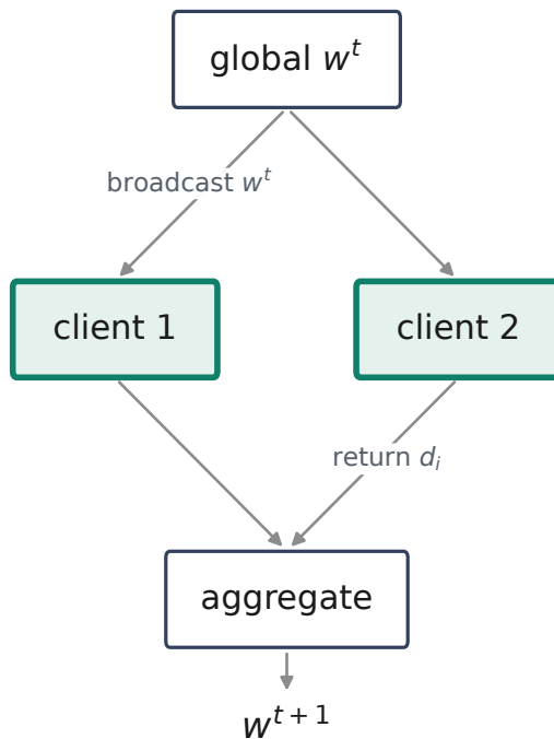
(b) FedProx
