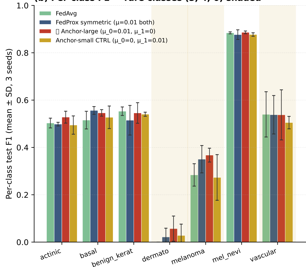
(b) Per-class F1 — rare classes (3, 4, 6) shaded
