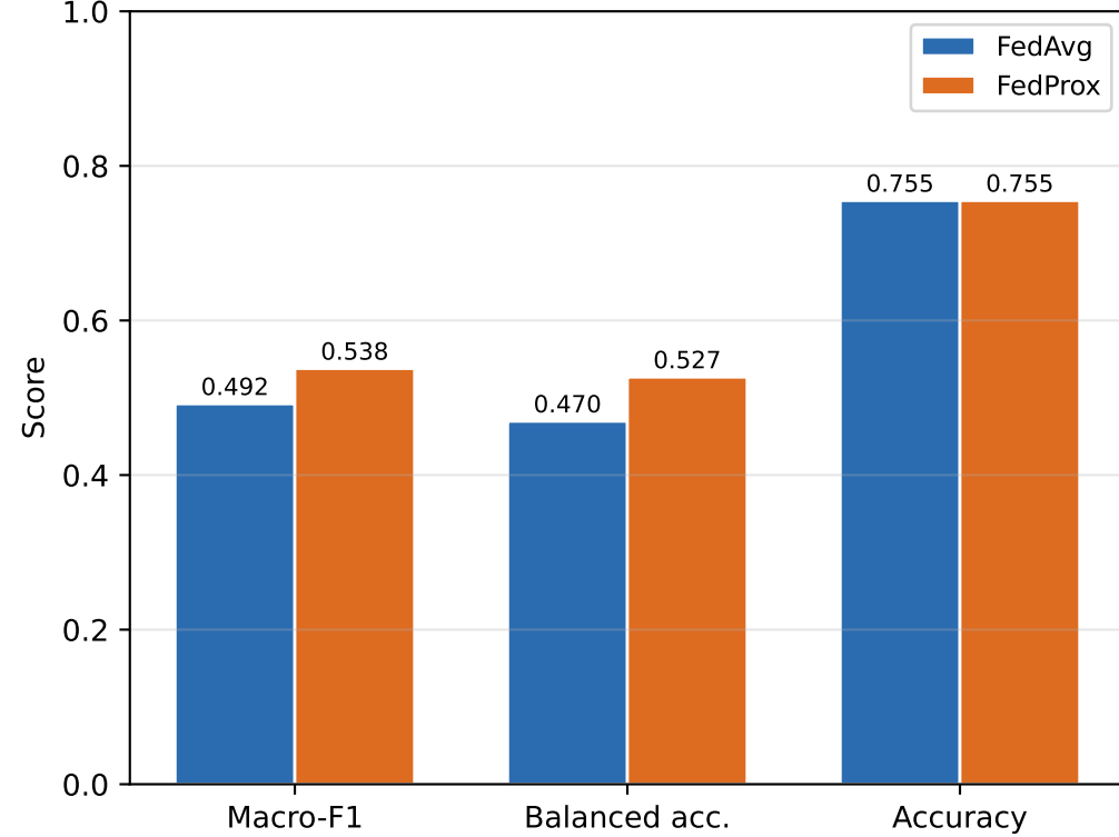
(D) Final test metrics
