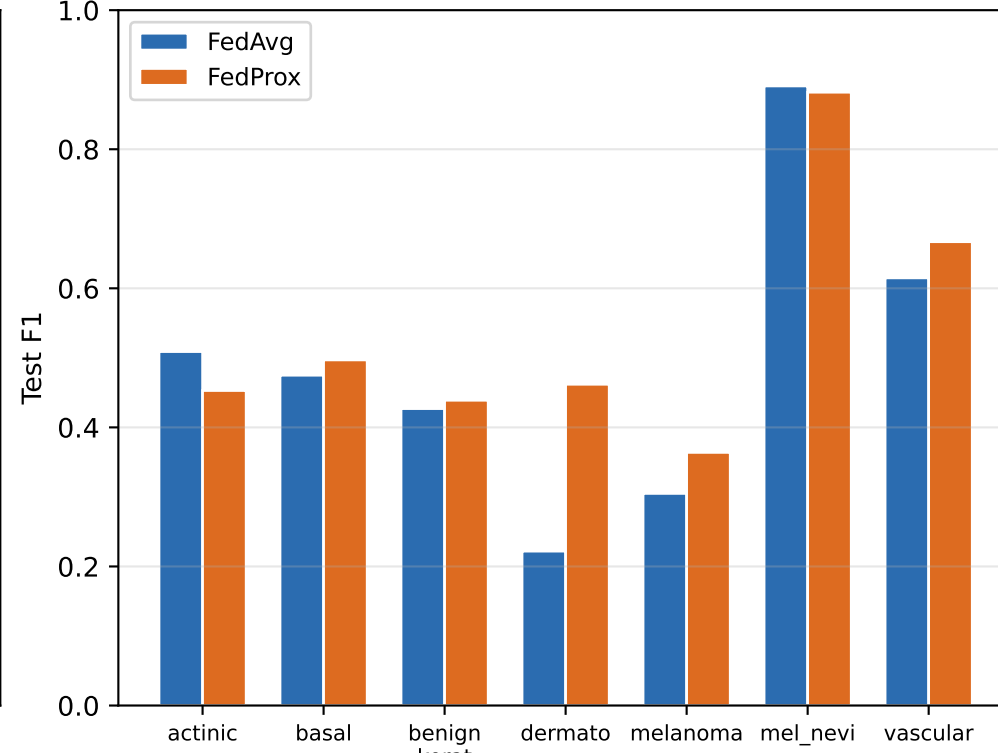
(E) Per-class test F1
