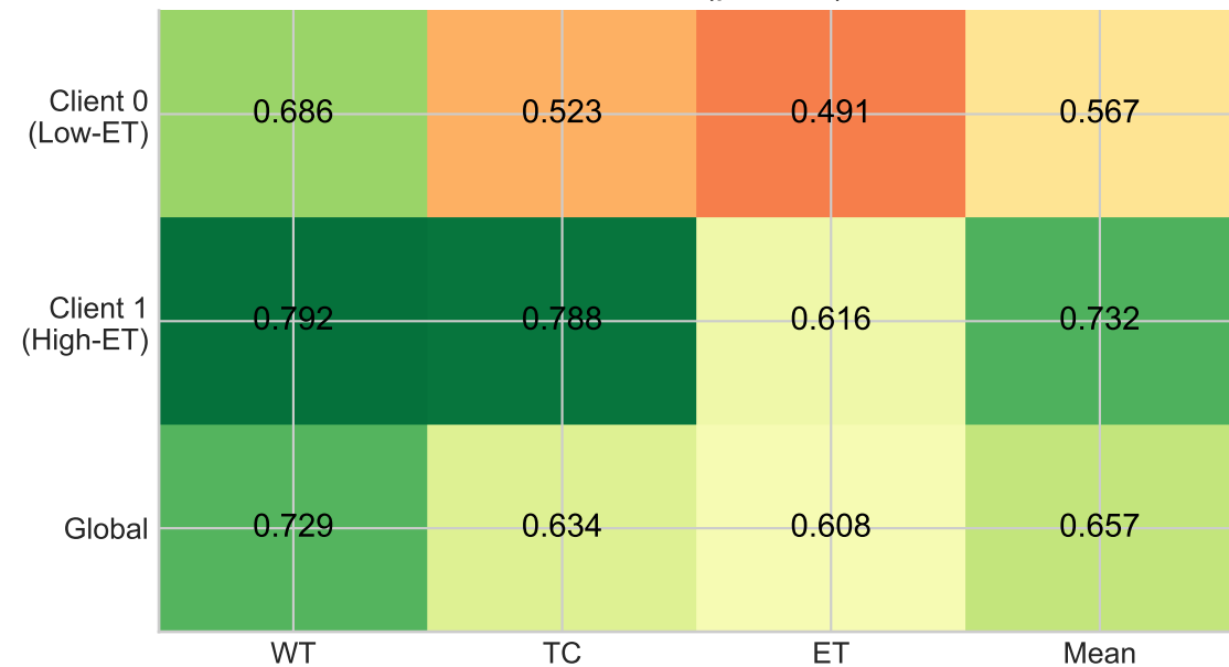
FedProx ( \mu=0.01 )
