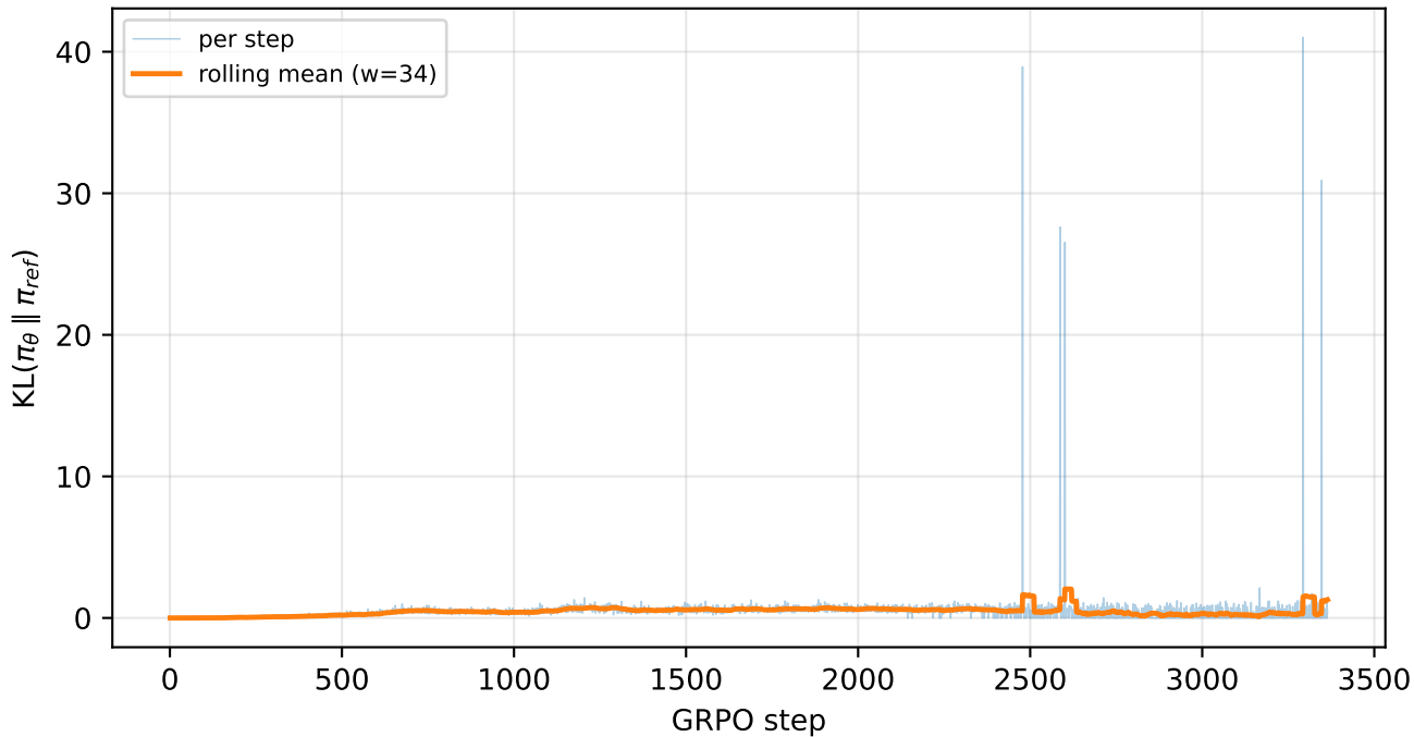
Baseline KL divergence (run jgs4c6kl)
