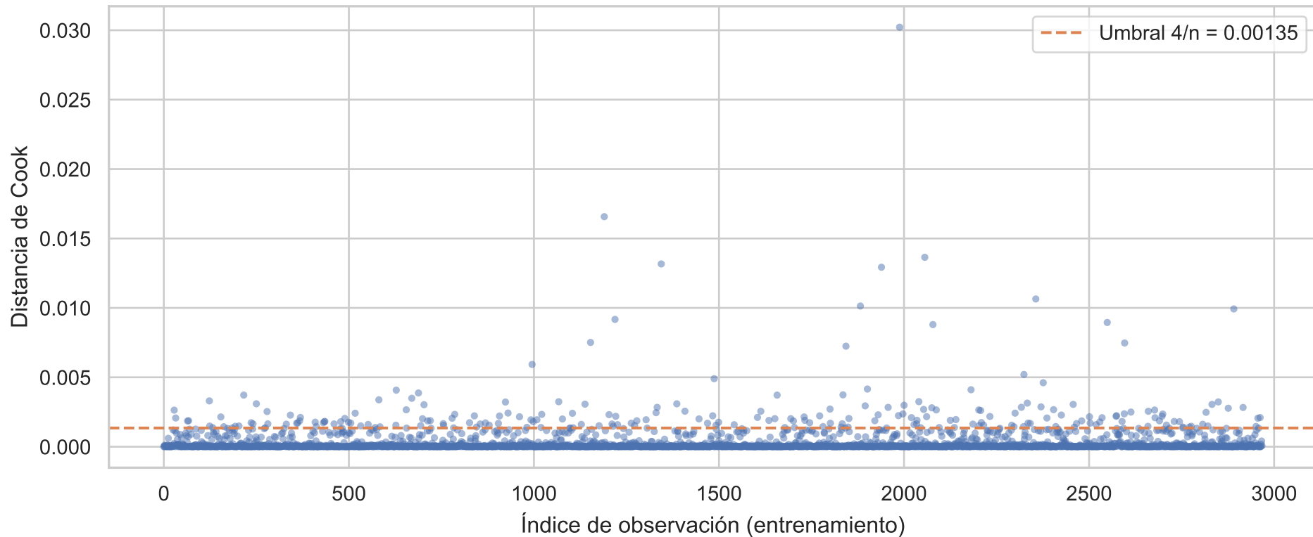
Observaciones influyentes — modelo final
