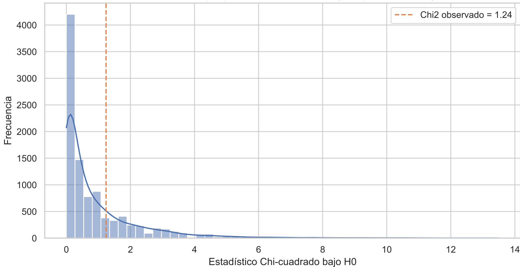
Distribución nula por permutación — Prueba 2 (tabaquismo vs. CHD)
