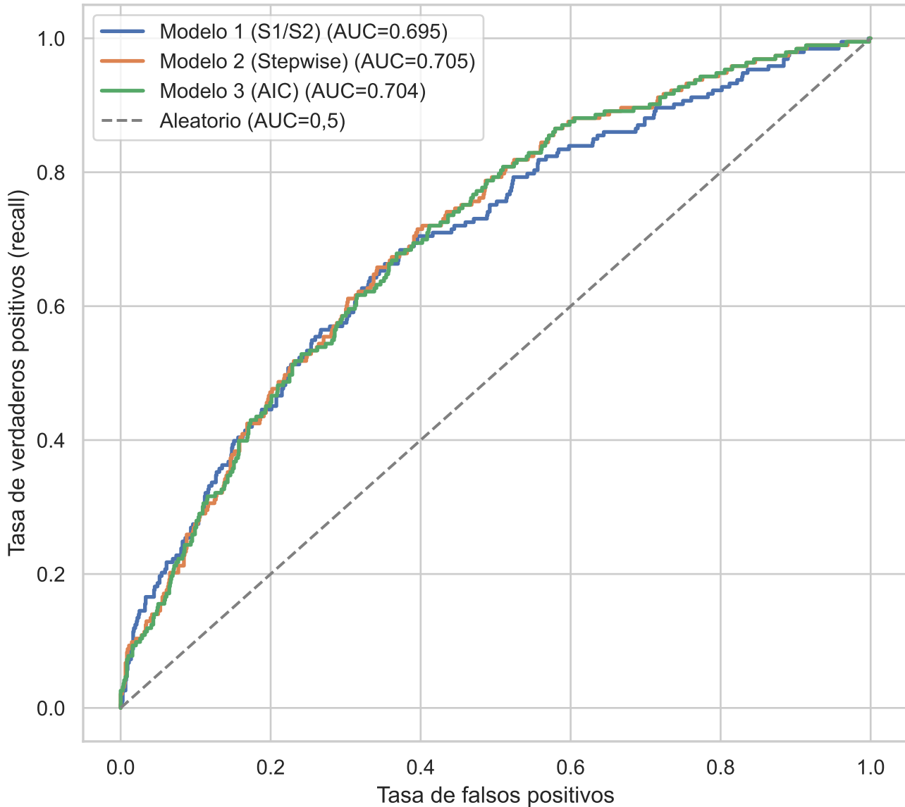
Curvas ROC — los 3 modelos, conjunto de prueba
