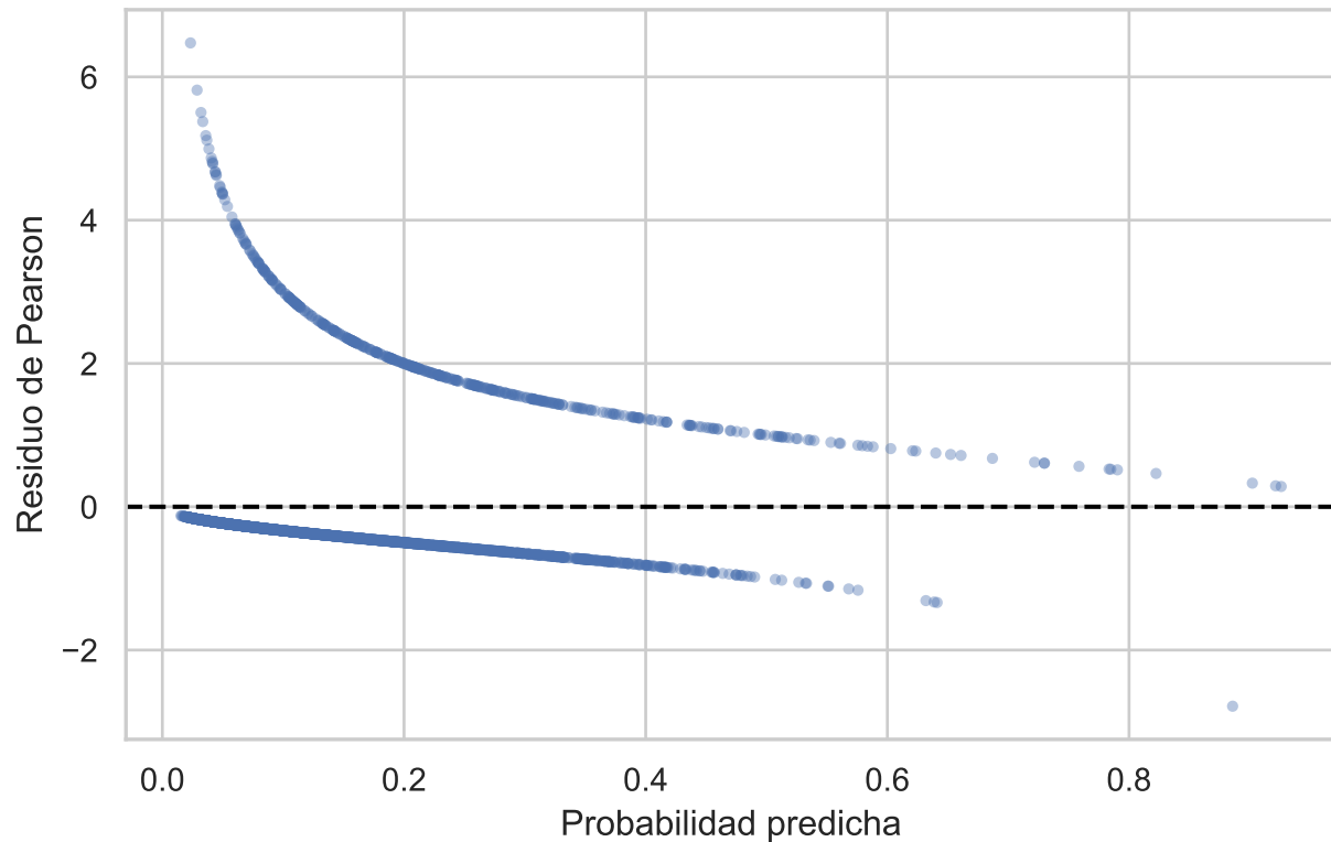
Residuos de Pearson vs. valores ajustados
