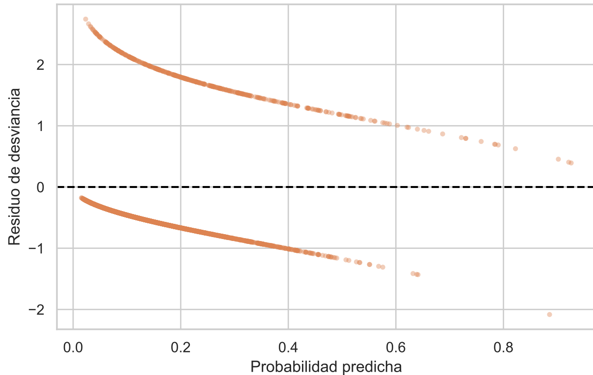
Residuos de desviación vs. valores ajustados
