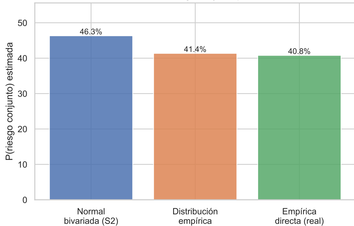
Estimación del riesgo conjunto por método
