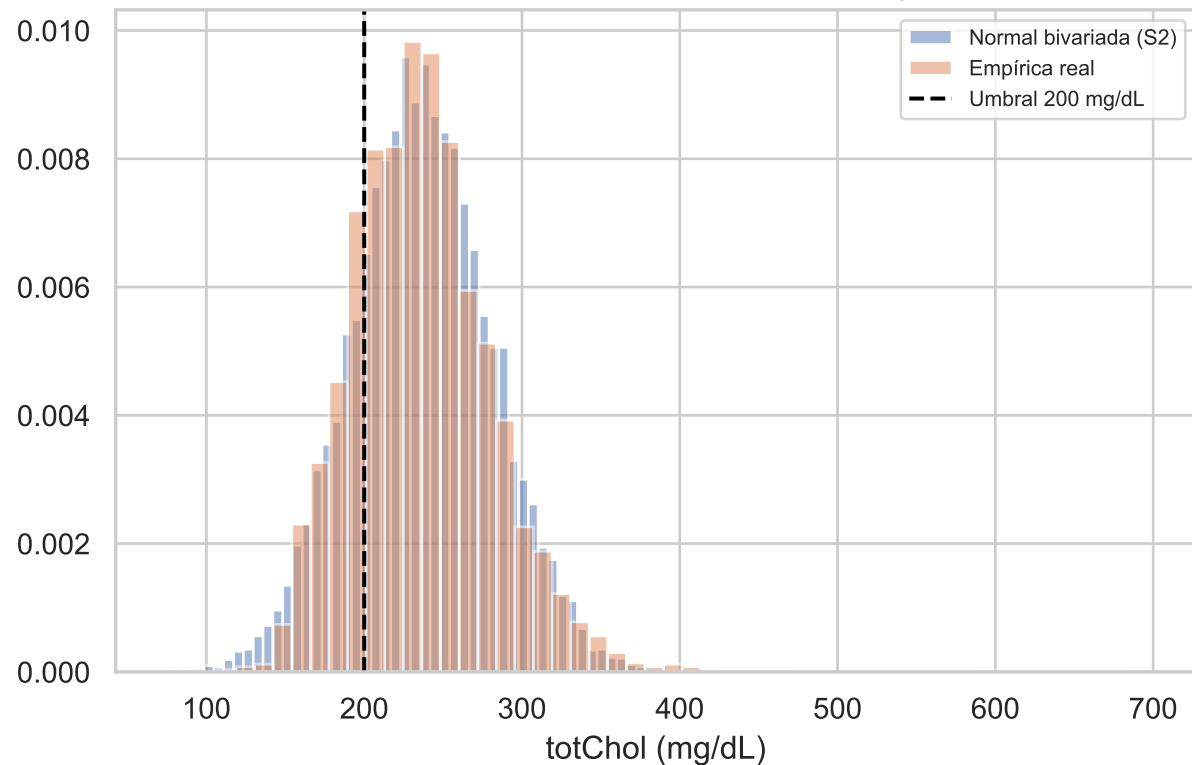
Cola derecha de totChol: normal vs. empírica
