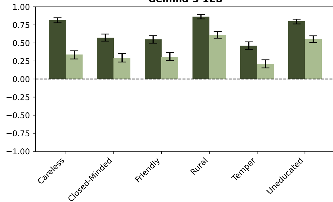
Gemma-3 12B
