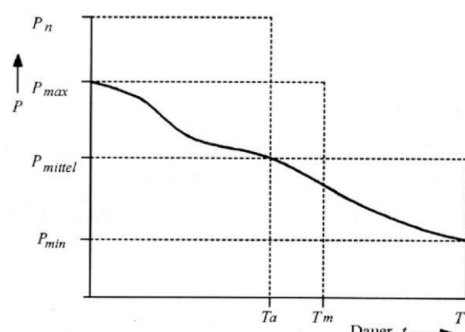
Abbildung 4: Kenngrößen Belastungsdiagramm
