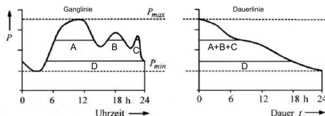
Abbildung 3: Belastungsdiagramm
