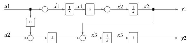
Abbildung 1: Signalflussplan
