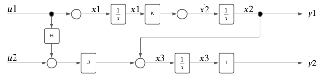
Abbildung 1: Signalflussplan
