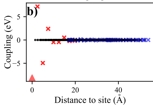
Zigzag
