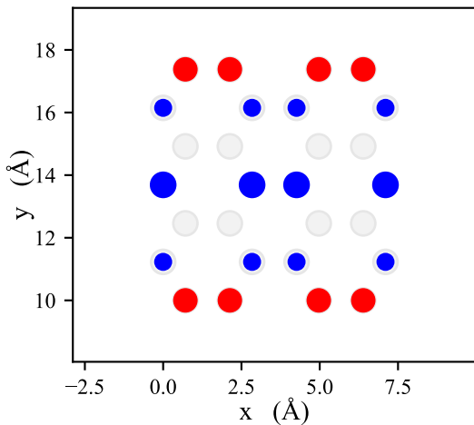
a-GNR, E=0.0 eV
