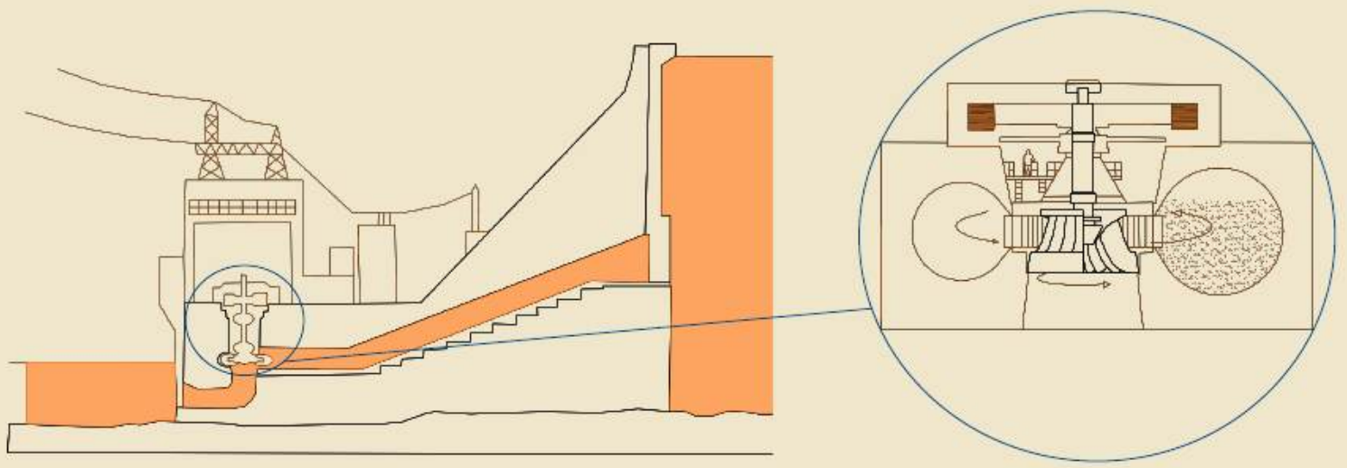
Centrale hydroélectrique, schématisation en coupe
