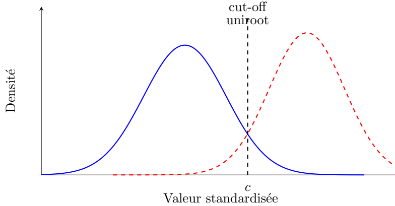
FIGURE 2 – Illustration de la méthode uniroot . La courbe bleue représente la population négative et la courbe rouge la population positive. Le seuil c correspond au point d'intersection entre les deux composantes gaussiennes estimées par le modèle de mélange.
