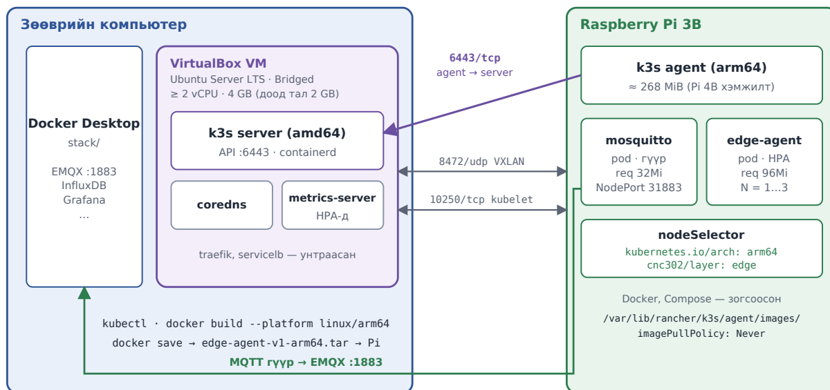
Зураг 8.2 — K3s кластер: зөөврийн компьютер дээрх VM (server, amd64) ба Raspberry Pi 3B (agent, arm64); портууд 6443/tcp, 8472/udp, 10250/tcp
