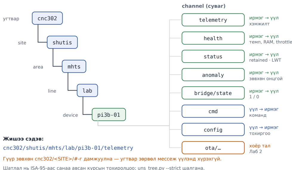
Зураг 3.2 — Unified Namespace-ийн шатлал: cnc302 / site / area / line / device / channel
