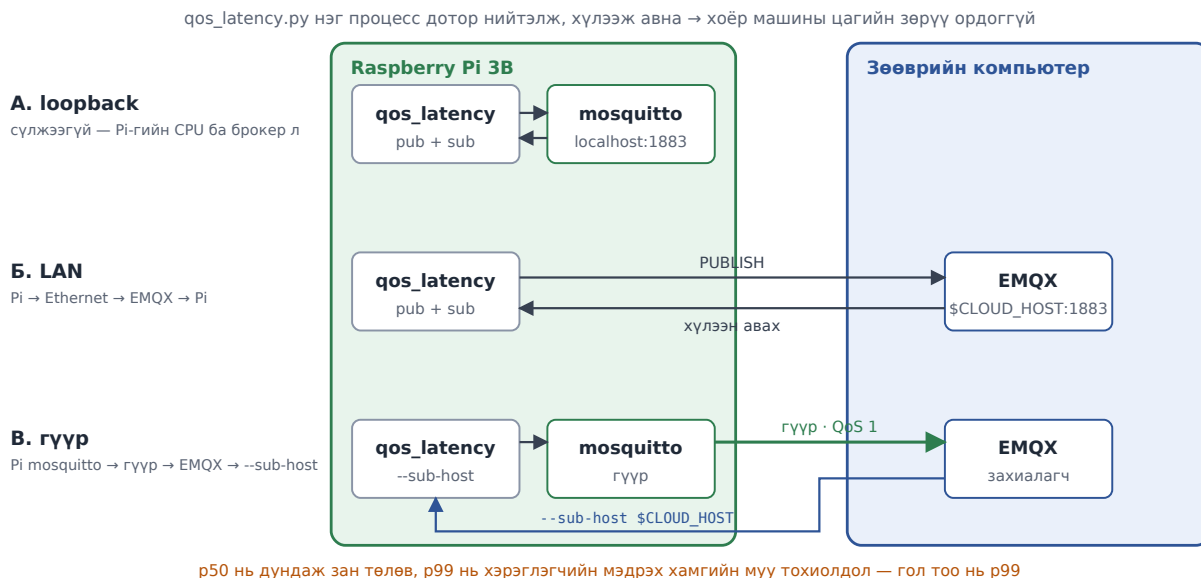
Зураг 1.2 — Саатлын гурван зам: loopback, LAN, гүүр
