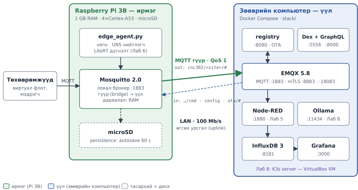
Зураг 0.1 — Хоёр давхаргат архитектур: зөөврийн компьютер (үүл) ба Raspberry Pi 3B (ирмэг), хооронд нь MQTT гүүр
