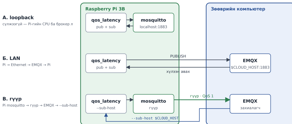
Зураг 3.3 — Хэмжилтийн гурван зам: loopback, LAN, гүүр
