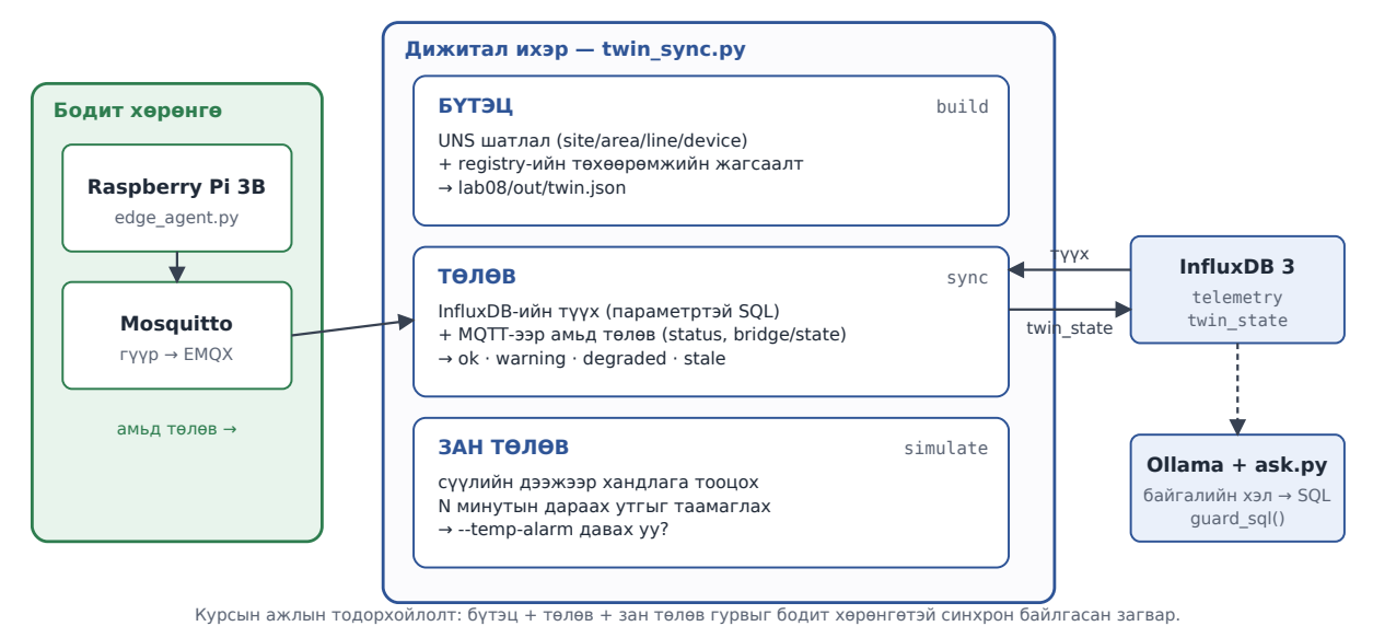
Зураг 8.1 — Дижитал ихрийн гурван давхарга: бүтэц (UNS + бүртгэл), төлөв (InfluxDB + гүүрээр ирэх амьд төлөв), зан төлөв (симуляц)
