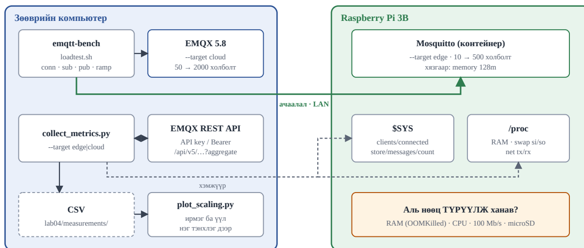
Зураг 4.1 — Ачааллын туршилтын бүтэц: emqtt-bench (зөөврийн компьютер) → ирмэгийн Mosquitto (Pi 3B) ба үүлний EMQX, хэмжүүр цуглуулалт
