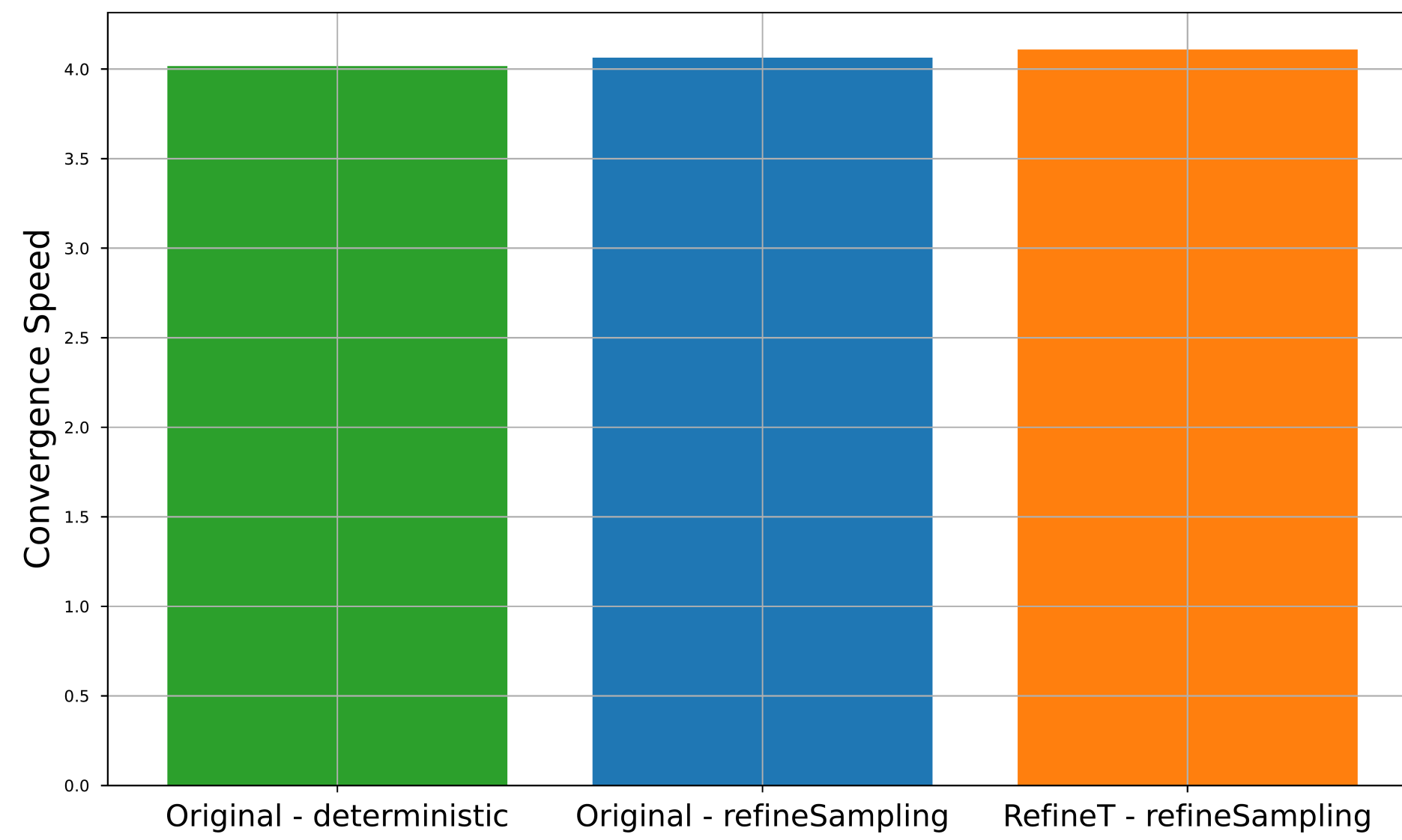
(d) Walker2d-v4
