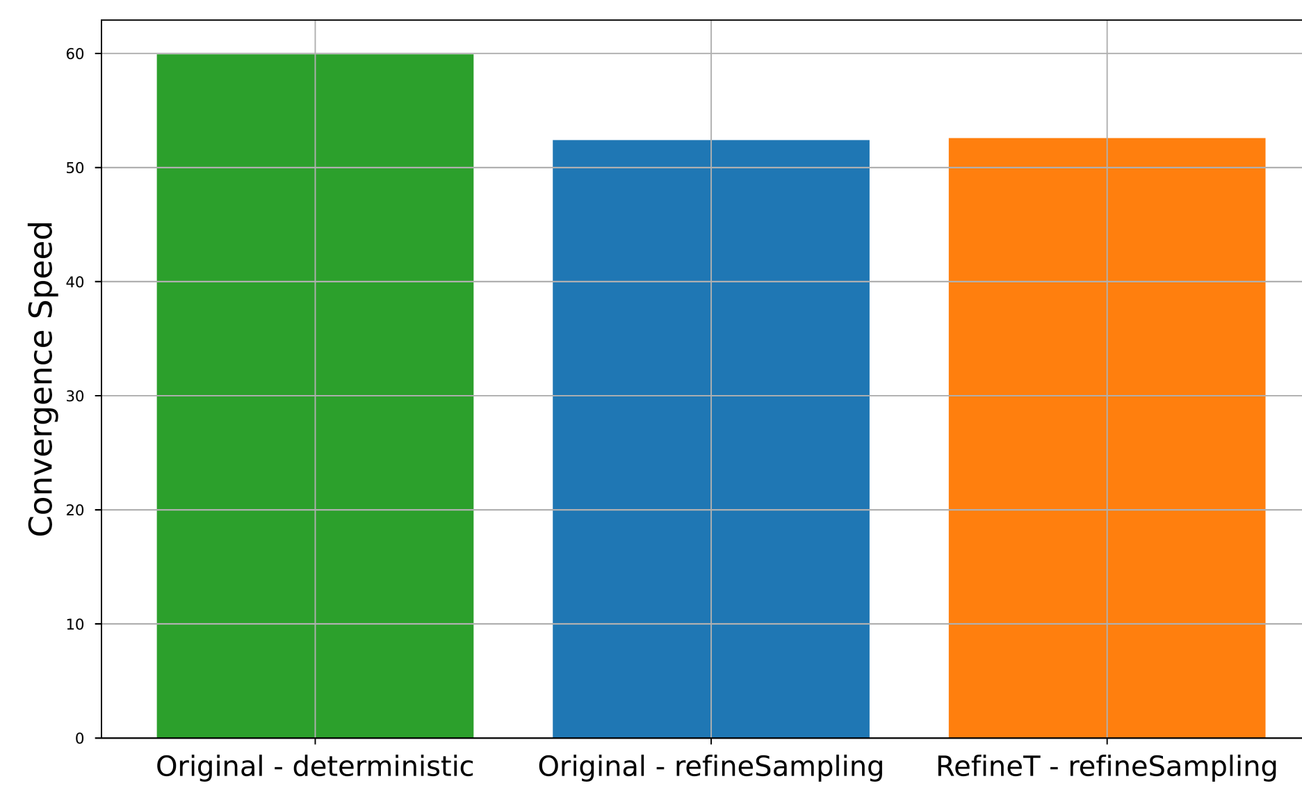
(b) HumanoidStandup-v4
