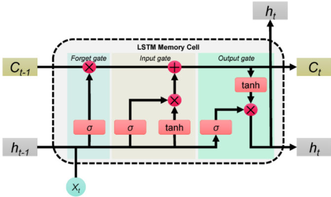
Abbildung 2.9.: Aufbau einer LSTM-Zelle: Der Zellzustand C_t wird durch Forget-, Input- und Output-Gate gesteuert, die per \sigma - und tanh-Aktivierung festlegen, was aus dem Gedächtnis verworfen, neu geschrieben und ausgelesen wird [16].
