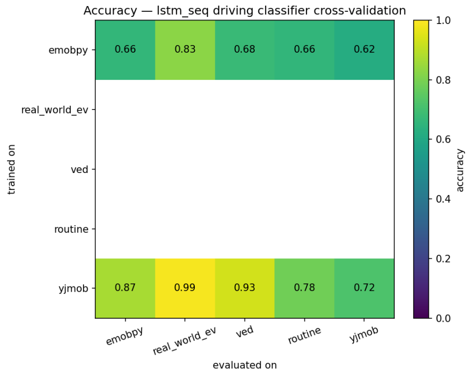
Abbildung A.7.: 5 \times 5 -Kreuzvalidierungsmatrix (Accuracy) des Driving-Classifiers (LSTM, sequenzielle Repräsentation)
