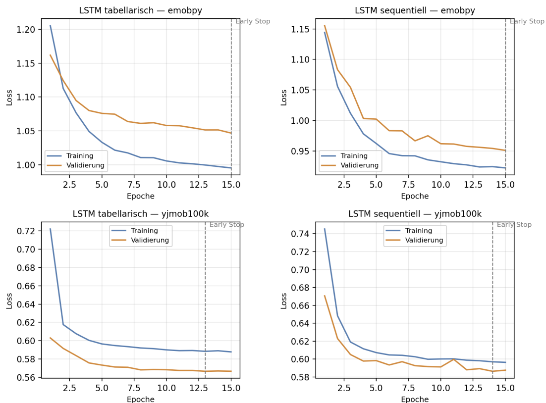
Abbildung 5.3.: Trainingskurven der LSTM-Varianten (tabellarisch und sequenziell) auf den zulässigen Datenquellen. Die gestrichelte Linie markiert den Haltepunkt, der durch Early Stopping Overfitting verhindert.
