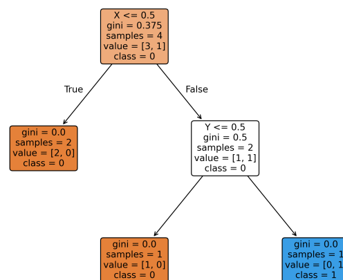
Abbildung 2.4.: Entscheidungsbaum mit Aufteilungskriterien (nach [10]).
