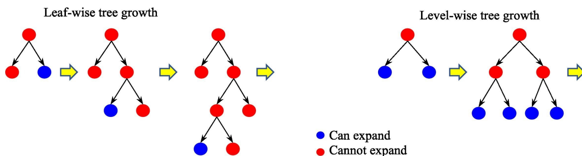
Abbildung 2.7.: Baumwachstum in Ensemble-Verfahren [13].
