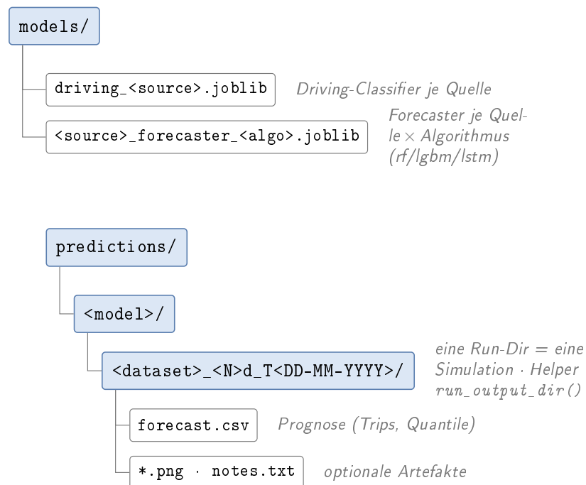
Abbildung 4.3.: Persistenzlayout
