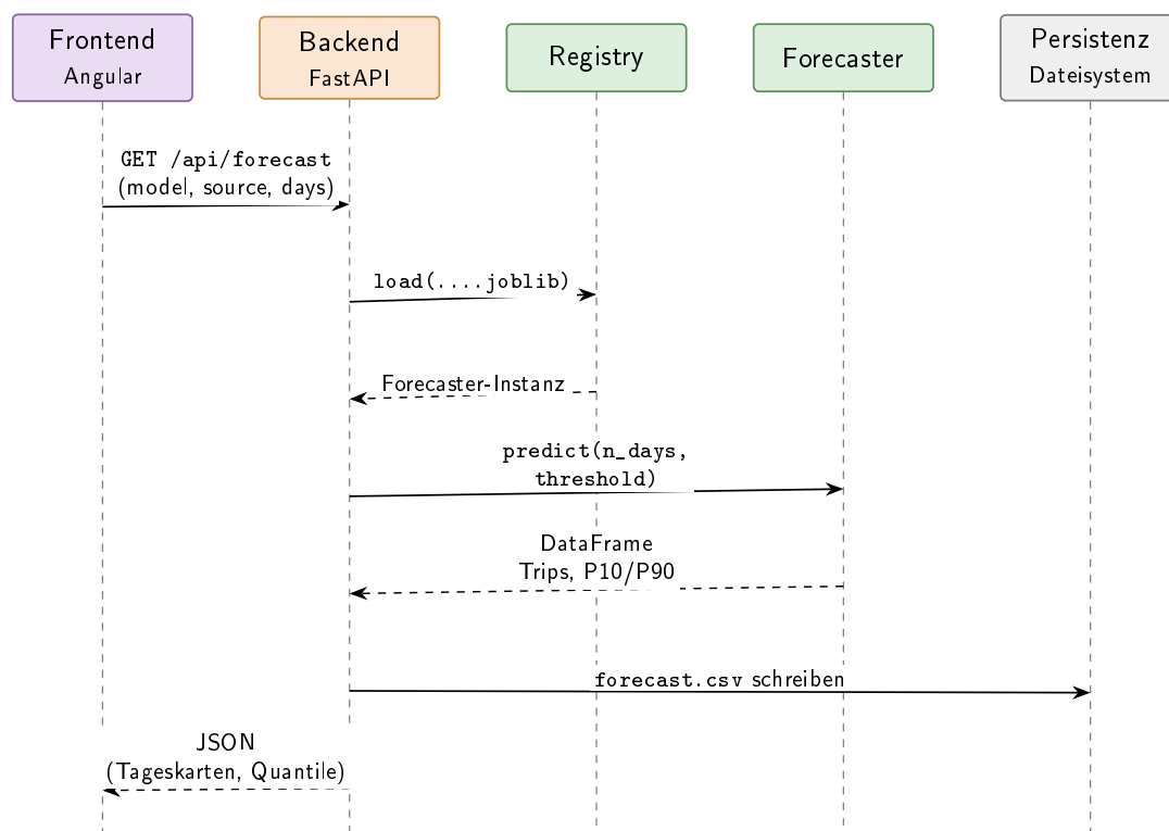
Abbildung 4.2.: Dynamischer Ablauf eines Forecast-Requests
