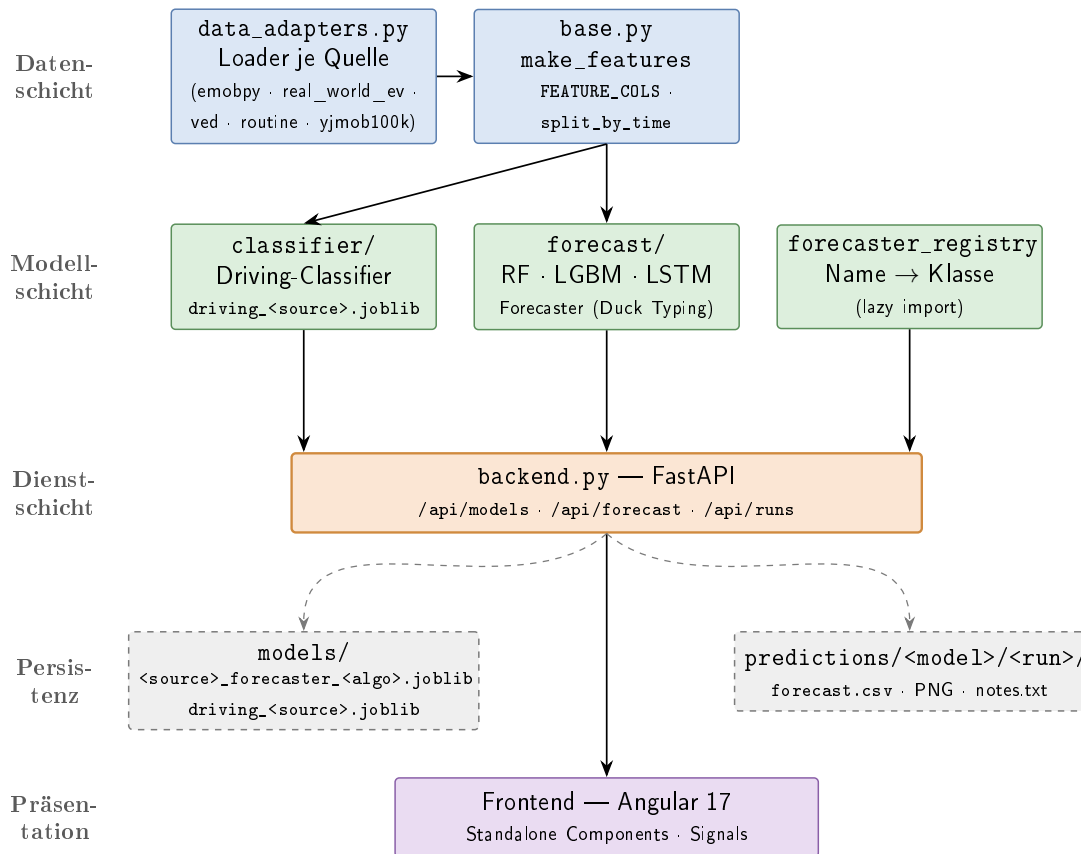
Abbildung 4.1.: Statische Komponentenstruktur
