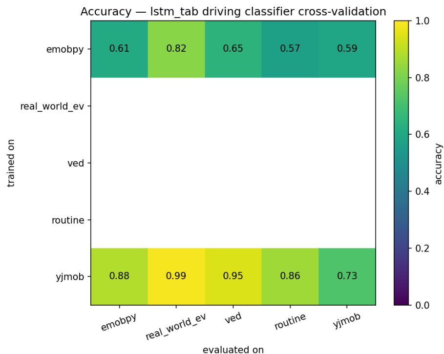
Abbildung A.6.: 5×5-Kreuzvalidierungsmatrix (Accuracy) des Driving-Classifiers (LSTM, tabellarische Repräsentation)
