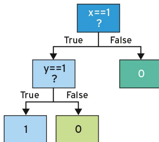
Abbildung 2.3.: Simpler binärer Entscheidungsbaum (Quelle: Schilli 2017).
