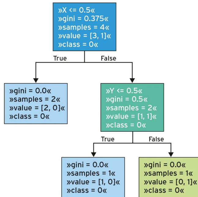
Abbildung 2.4.: Entscheidungsbaum mit Aufteilungskriterien (Gini-Index, Stichprobengröße und Klassenverteilung pro Knoten) (Quelle: Schilli 2017).
