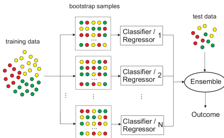
Abbildung 2.4.: Bagging: Aus den Trainingsdaten werden N Bootstrap-Stichproben gezogen, auf denen jeweils ein Baum trainiert wird; deren Vorhersagen werden zu einem Ensemble aggregiert (ResearchGate 2022).
