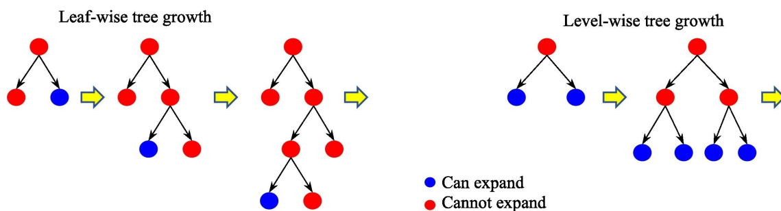
Abbildung 2.6.: Baumwachstum in Ensemble-Verfahren (ScienceDirect 2026).
