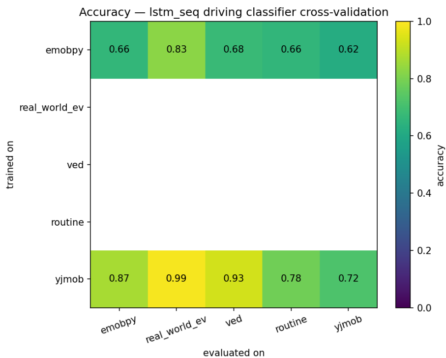
Abbildung A.7.: 5 \times 5 -Kreuzvalidierungsmatrix (Accuracy) des Driving-Classifiers (LSTM, sequentielle Repräsentation)
