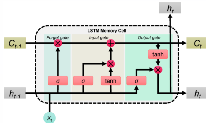
Abbildung 2.8.: Aufbau einer LSTM-Zelle: Der Zellzustand C_t wird durch Forget-, Input- und Output-Gate gesteuert, die per \sigma - und \tanh -Aktivierung festlegen, was aus dem Gedächtnis verworfen, neu geschrieben und ausgelesen wird (dida 2026).
