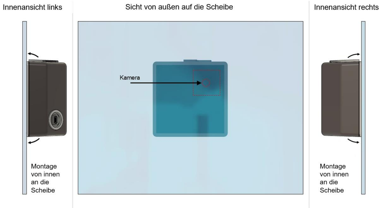
Abbildung: Ansichten des Geräts nach Montage durch Ankleben auf die Glasscheibe
