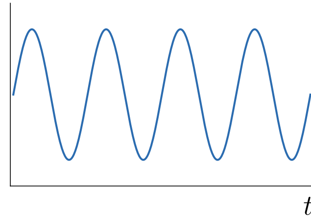
Periodic
