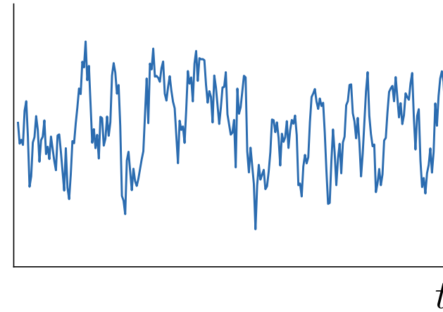
Autoregression
