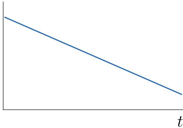
LocalTrend
