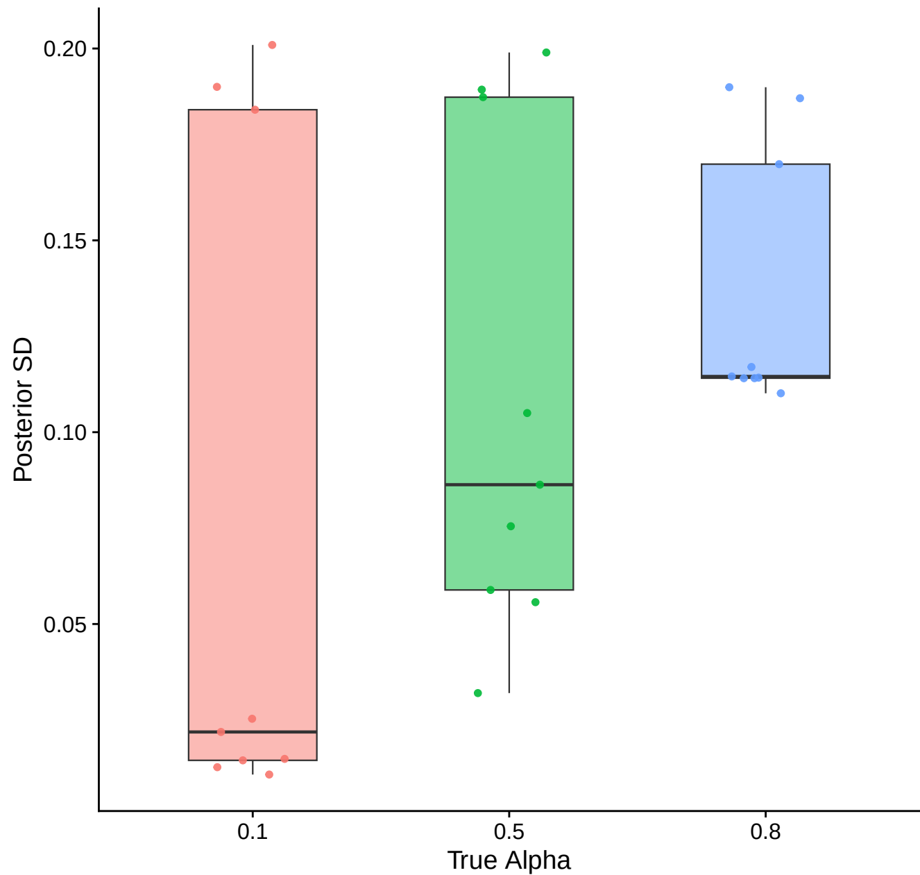
Posterior SD of Alpha
