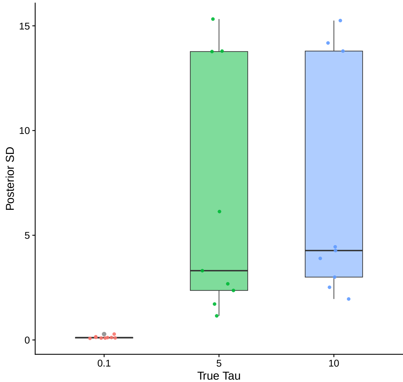
Posterior SD of Tau
