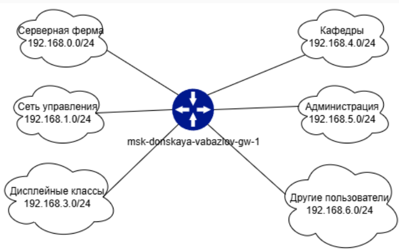
Рис. 5: L3 192.168.0.0/16
