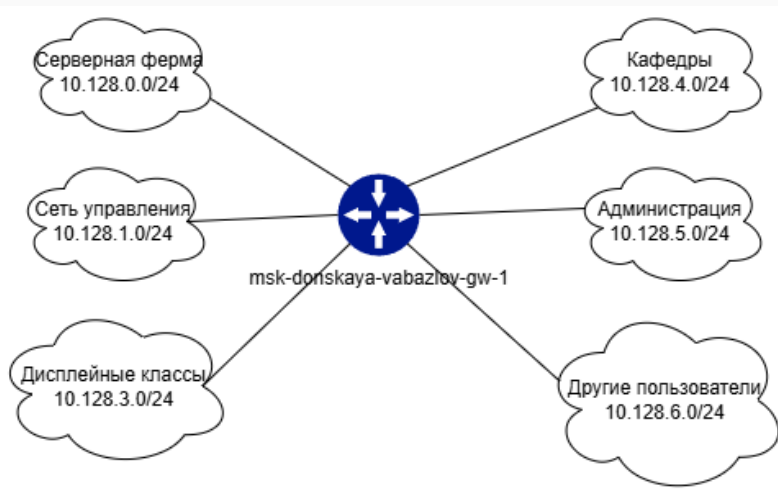
Рис. 3: Схема L3
