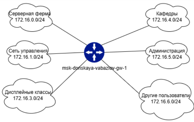
Рис. 4: L3 172.16.0.0/12
